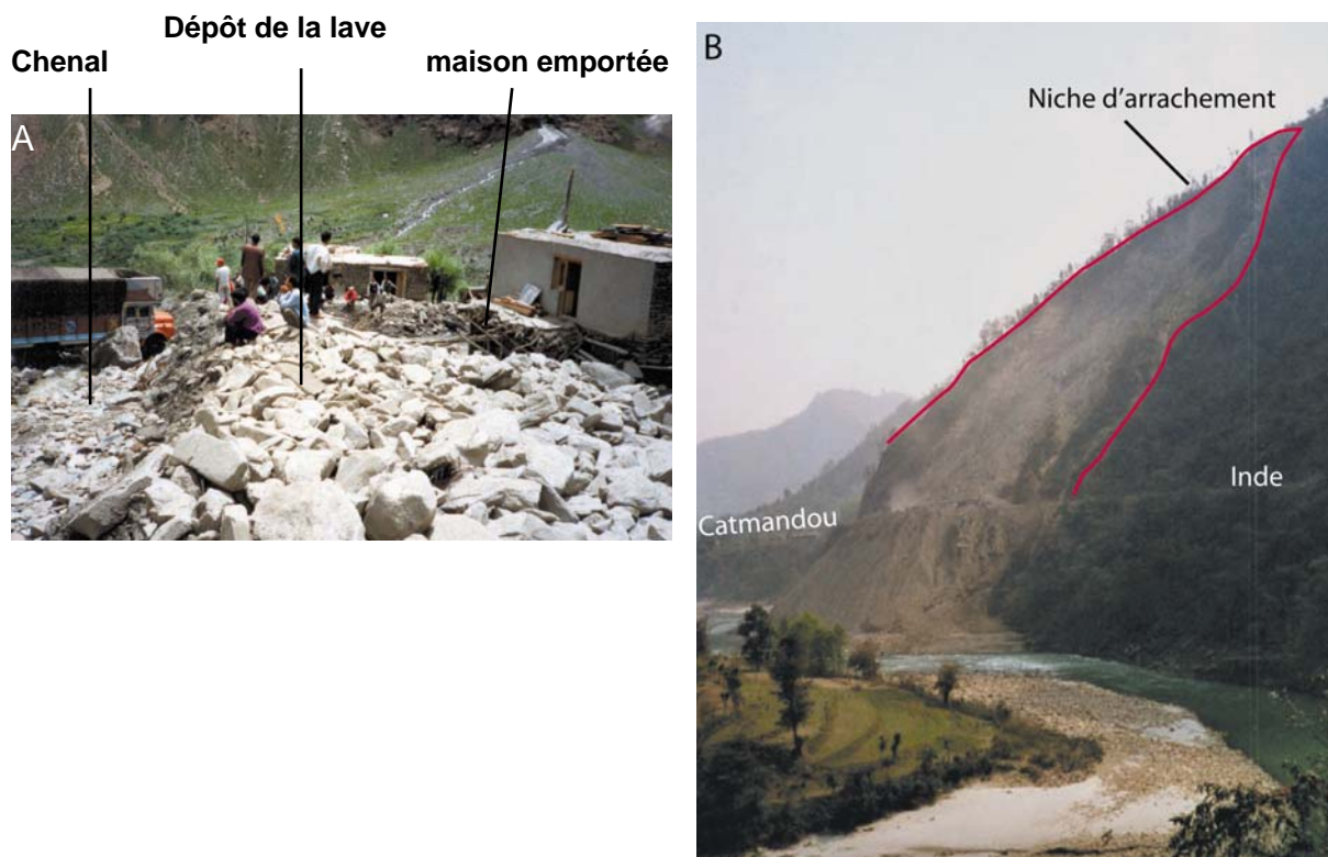
Figure 5 - Deux événements de coupure de route stratégique dans l'Himalaya. A : Lave torrentielle coupant la route transhimalayenne donnant d'accès au Cashmire indien (d'après [16]). B : Glissement de Krisnabir coupant la route d'accès à Katmandou depuis l'Inde.
